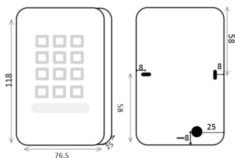
Wymiary w mm.
